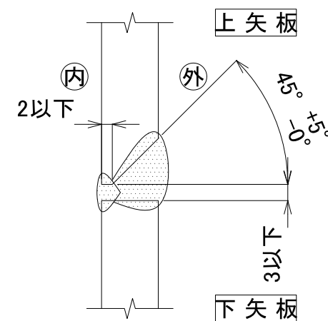
開先形状図 S=1/1
