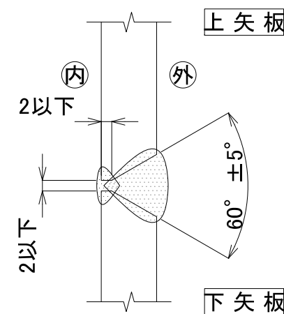
開先形状図 S=1/1
