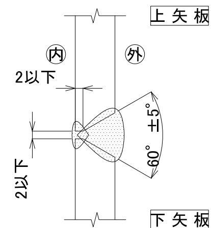
開先形状図
