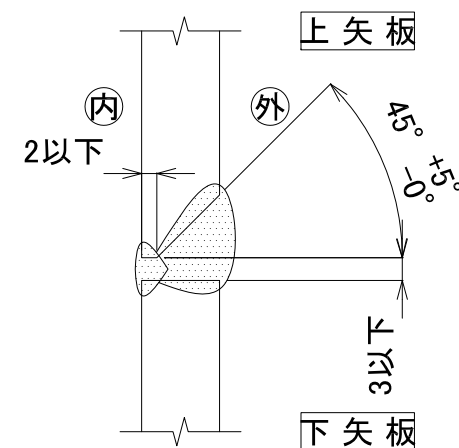
開先形状図
