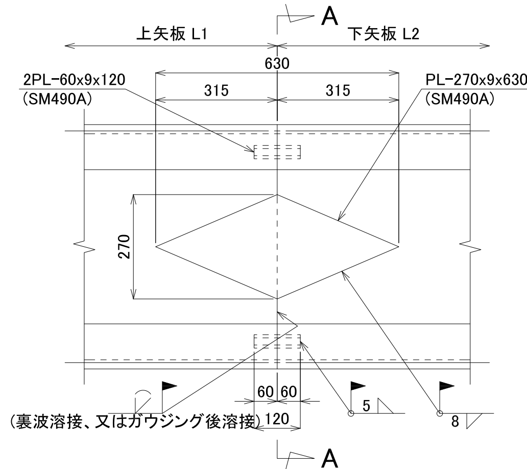
開先加工範囲
