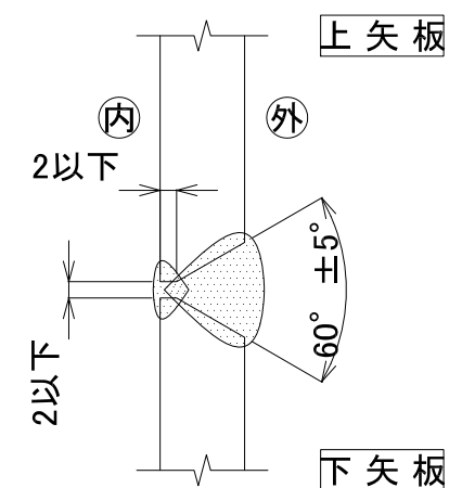
開先形状図 S=1/1
