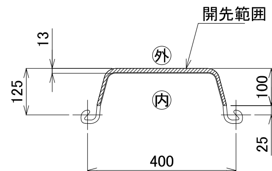
開先加工範囲
