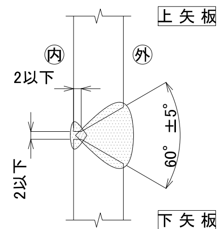
開先形状図 S=1/1
