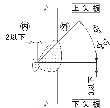
開先形状図
