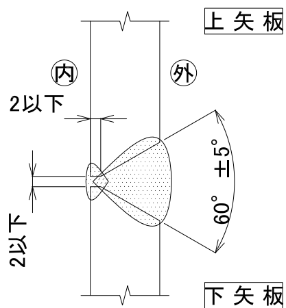
開先形状図
