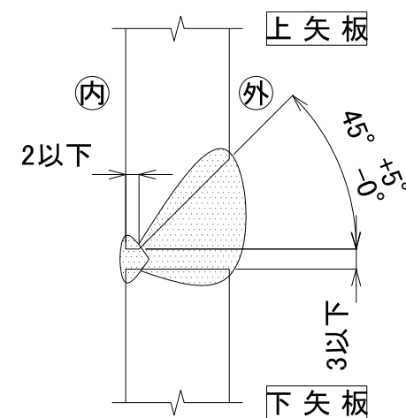
開先形状図 S=1/1
