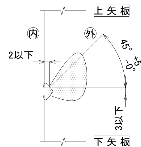
開先形状図
