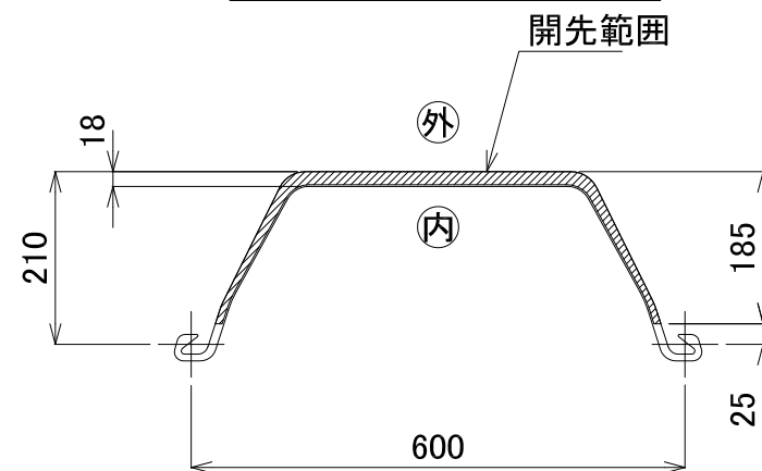
開先加工範囲
