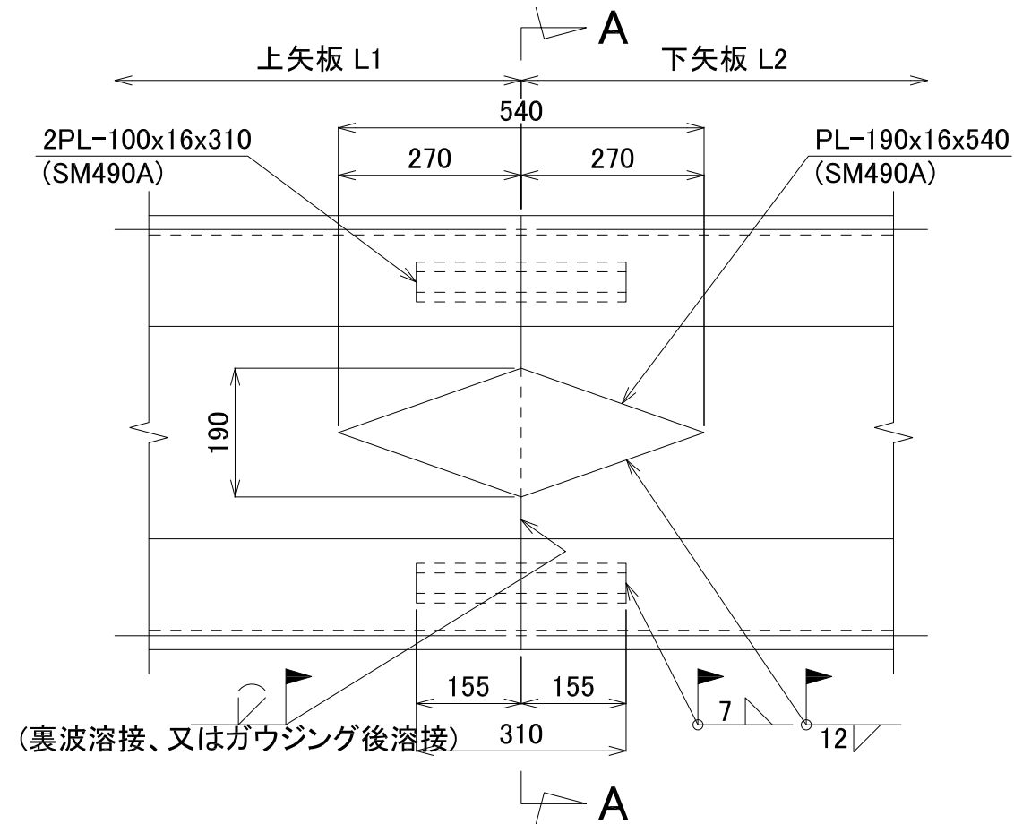
開先加工範囲
