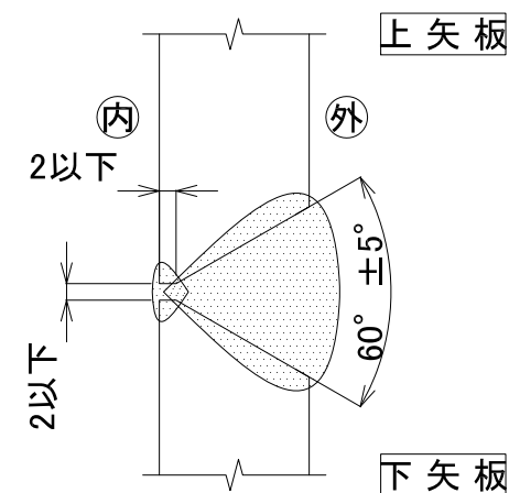
開先形状図
