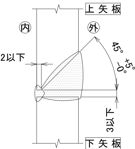
開先形状図
