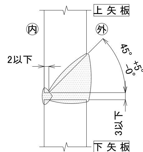
開先形状図 S=1/1
