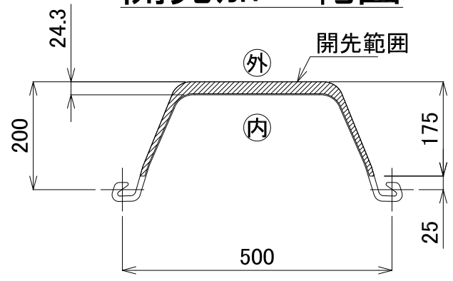
開先加工範囲
