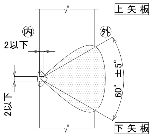
開先形状図 S=1/1
