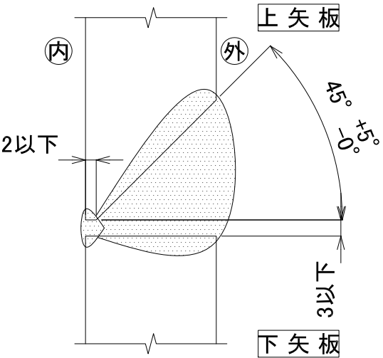
開先形状図 S=1/1
