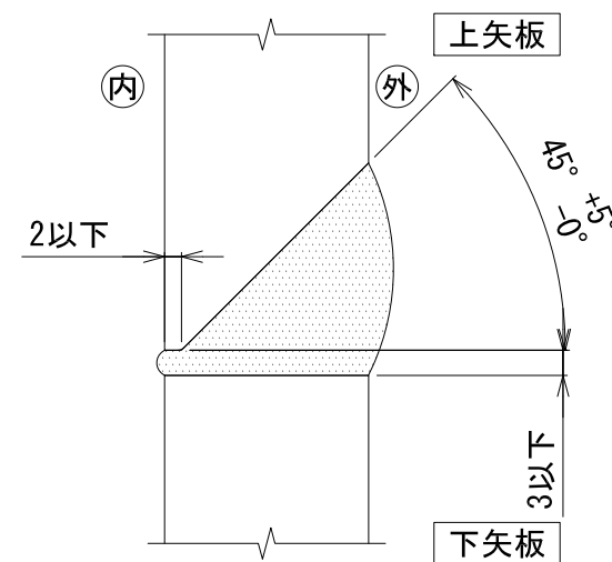
開先形状図
