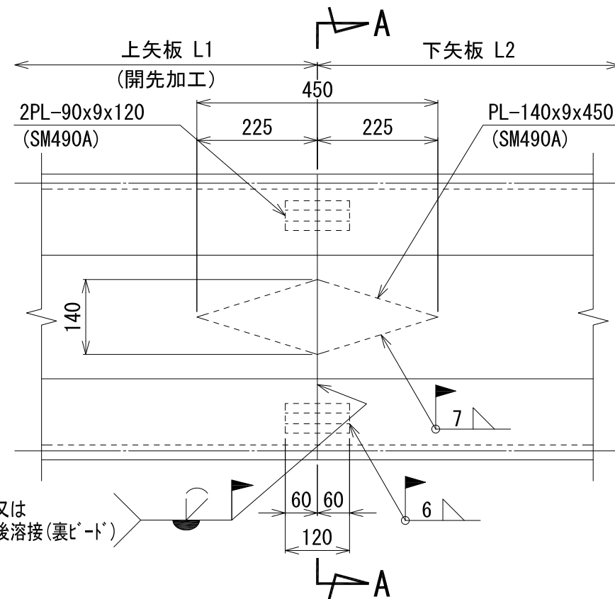
開先形状図
