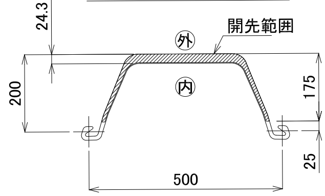
開先加工範囲
