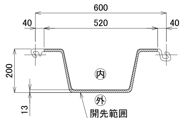
上矢板を下側(開先を取る側)からみた図
