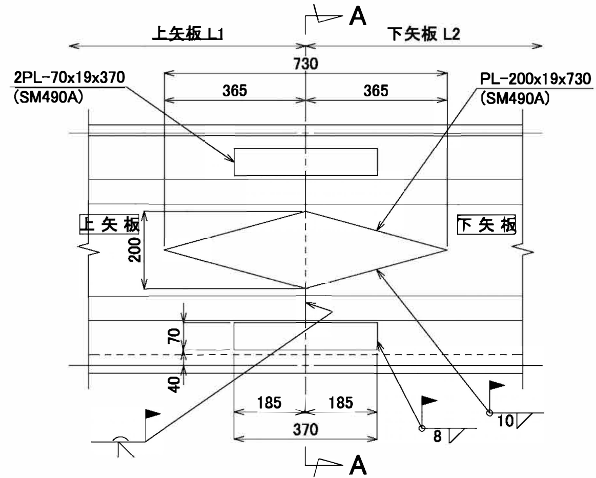
矢視 B-B
